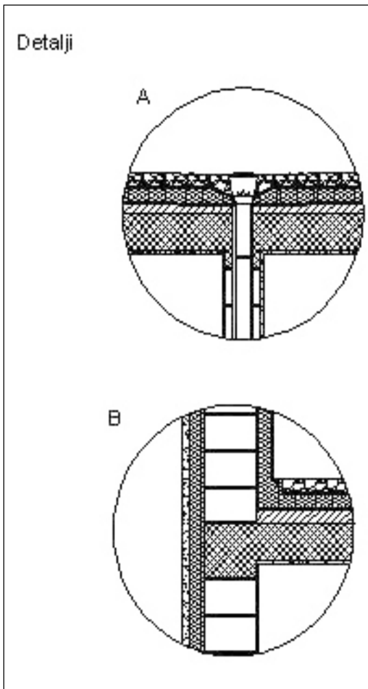
Detalji
