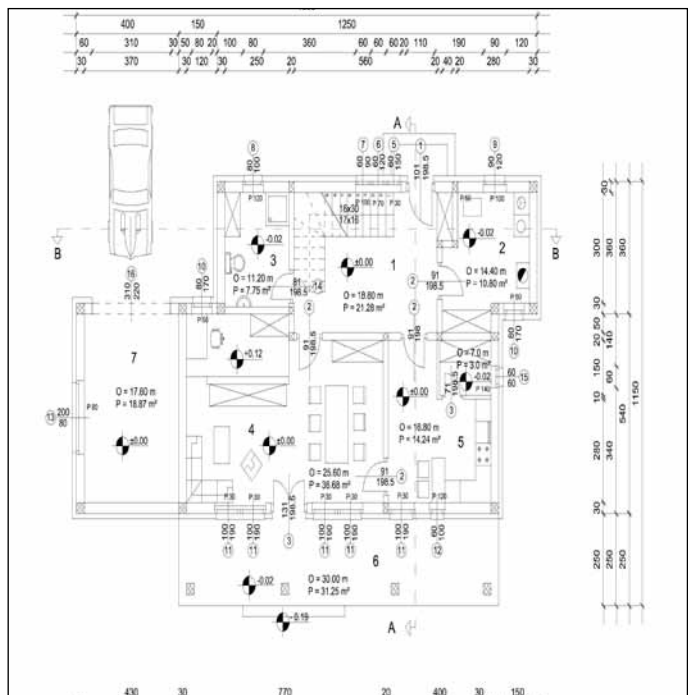
Tlocrt prizemlja - obiteljska kuća
