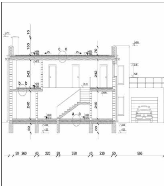
PRESJEK B-B- Obiteljska kuća
