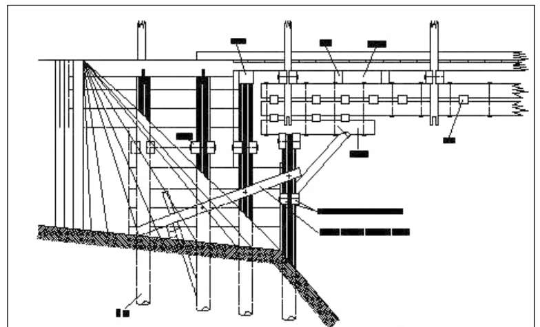
Upornjak s paralelnim krilima
