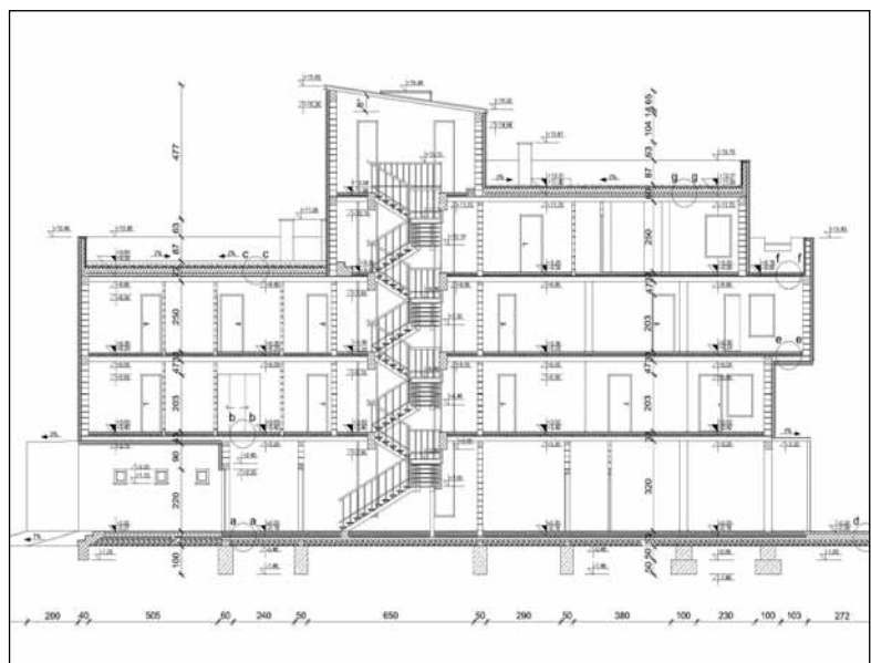
Presjek A-A- Stambeno poslovna zgrada
